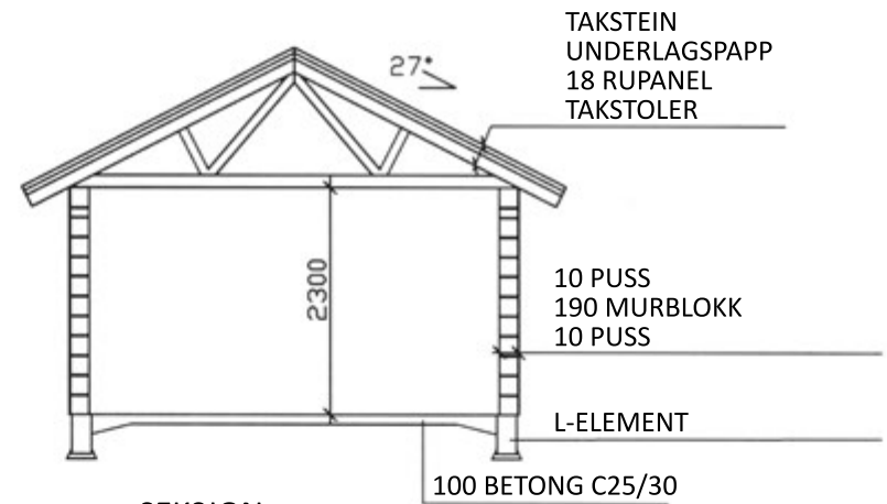
SEKSJON
