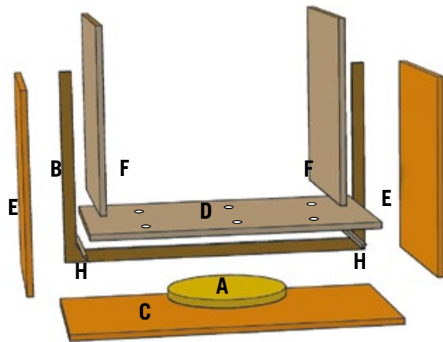
Skisse 1. Formens deler – før montering
